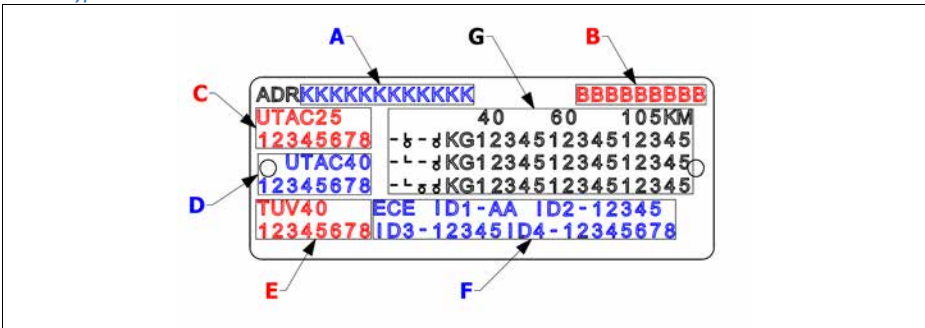
Achsenschild in Form eines Aufklebers
