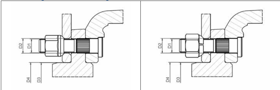
1. Einzelrad mit Mutter
