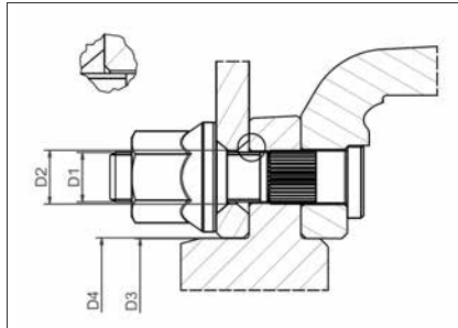
5. Einzelrad mit konischer Mutter
