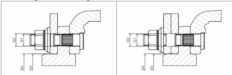
6. Einzelrad mit Mutter ISO
